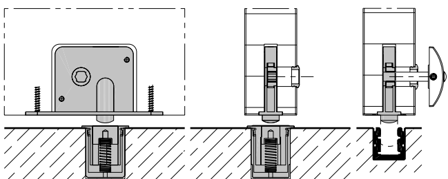
Fermeture dans douille de sol no 13787
