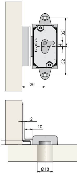
Technische tekening om te schroeven
