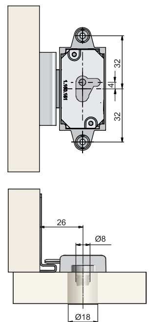
Technische tekening met drevels
