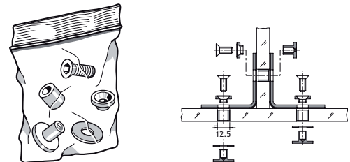
Bevestigingset hoek glas-glas voor winkelhaak.
