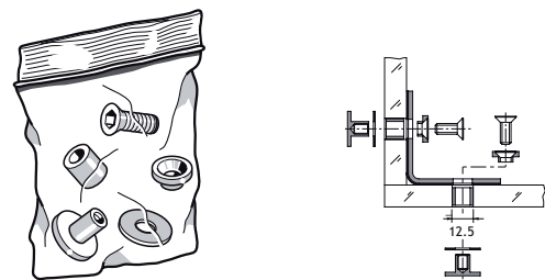
Bevestigingset glas-glas voor winkelhaak.
