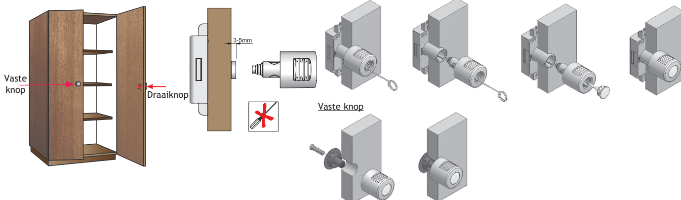
Toepassingsvoorbeeld
