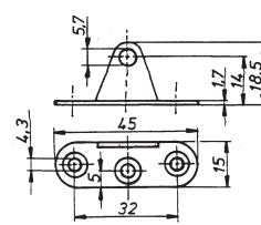
Compas d'abattant EXQUISIT MSE à frein à visser - SANS AIMANT
