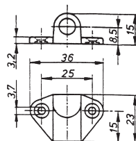
Compas d'abattant EXQUISIT MSE à frein à visser - SANS AIMANT
